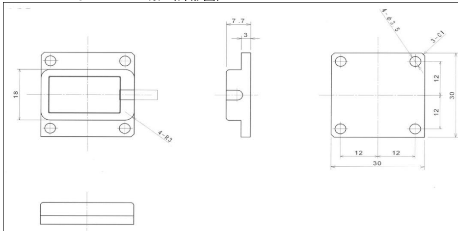
MA3-**BA-RDB※ (外形図)
